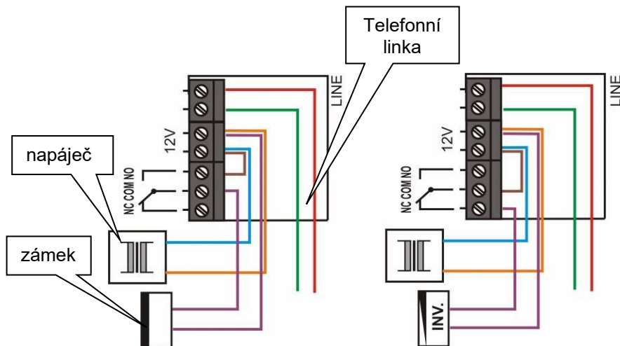
Připojení kabelů a zapojení standardního a inverzního zámku.
