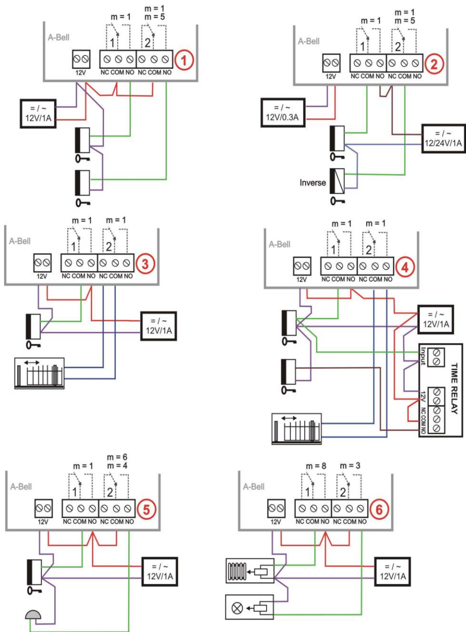
Obr. 3 Příklady zapojení spínačů
