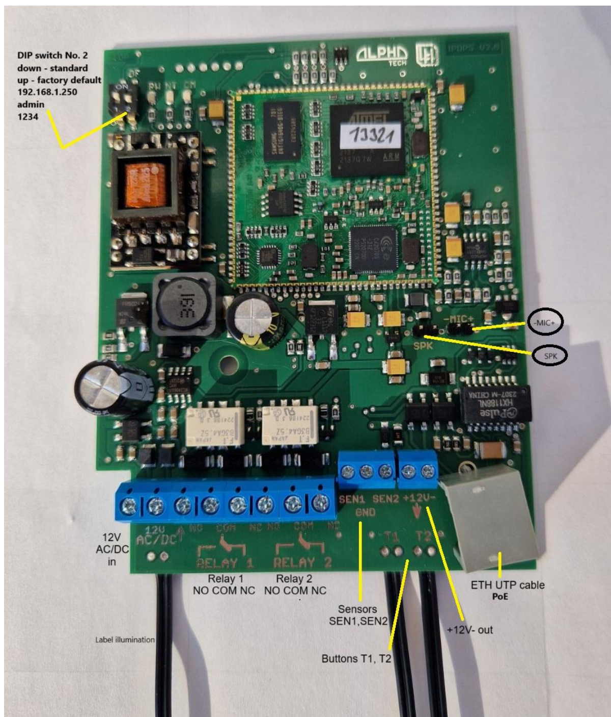
IP-Slim-audio-plošný-spoj-popis
